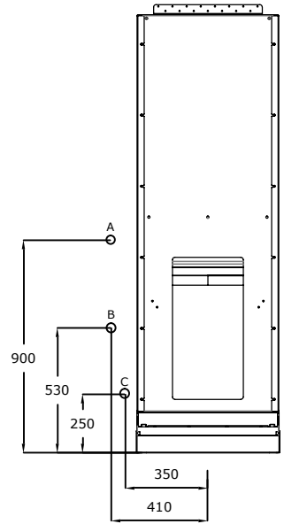
AANSLUITING OPTIE 2
