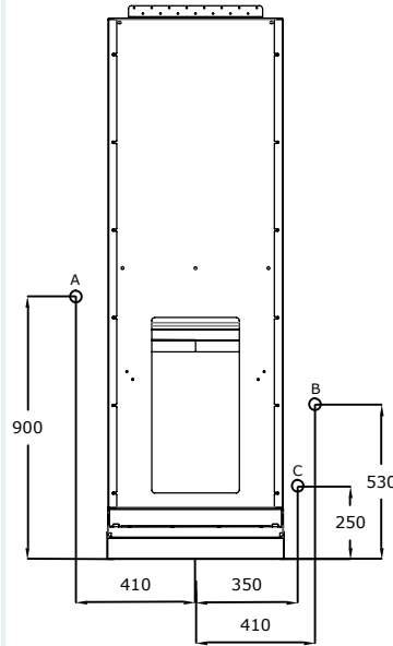
AANSLUITING OPTIE 1
